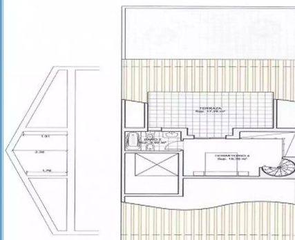
PLANTA BAJOCUBIERTA E: 1/100
