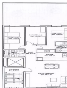
PLANTA SEGUNDA E: 1/100
